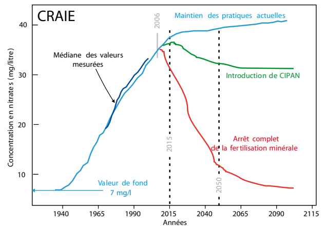
Figure 32 : Aquifère de la Craie : évolution comparée de la médiane des concentrations calculées pour chaque scénario (Laisser Faire, CIPAN, arrêt total de la fertilisation azotée).
