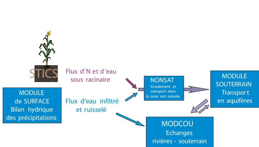
Figure 17 : Principe général du couplage STICS-MODCOU.
