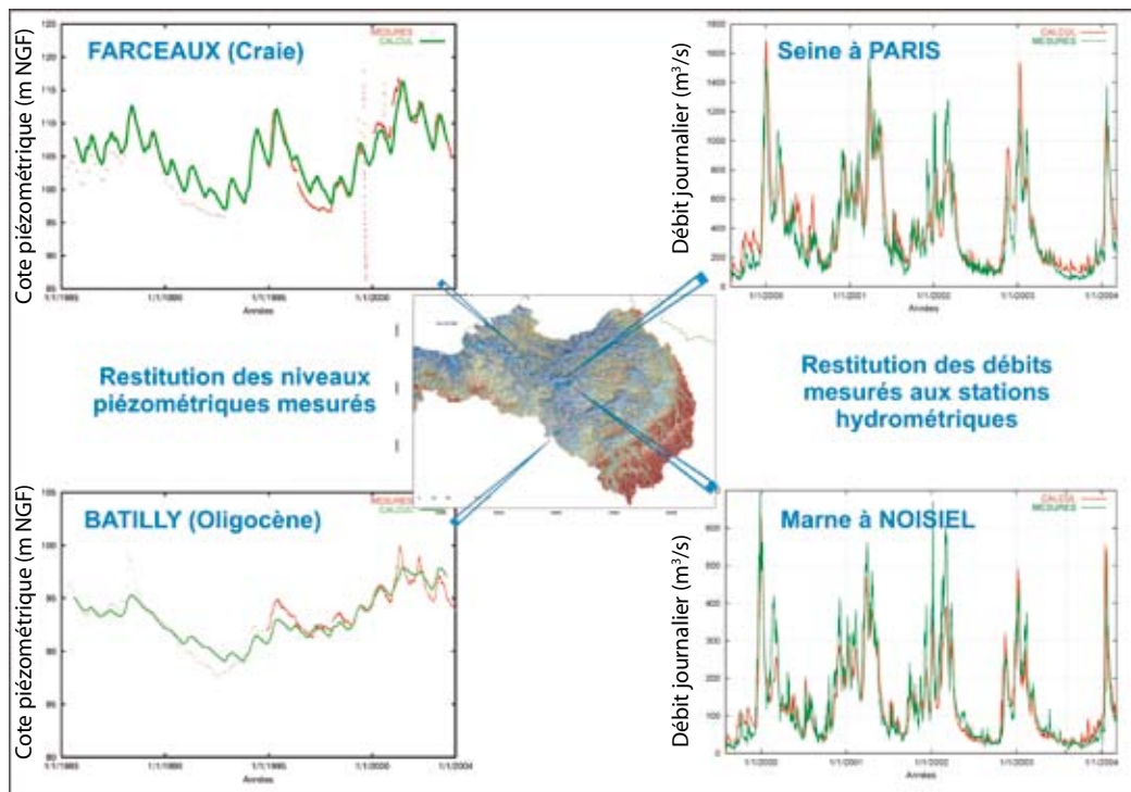
Figure 9 : Calage hydrodynamique du modèle en termes de restitution des cotes piézométriques des aquifères et de débit des rivières.
