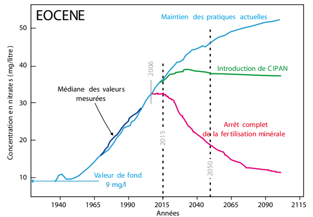
Figure 31 : Aquifère de l'Éocène : évolution comparée de la médiane des concentrations calculées pour chaque scénario (Laisser Faire, CIPAN, arrêt total de la fertilisation azotée).
