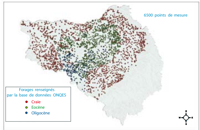
Figure 6 : Répartition géographique des forages de la base de données ONQES sur les aquifères de la Craie, de l'Eocène et de l'Oligocène.
