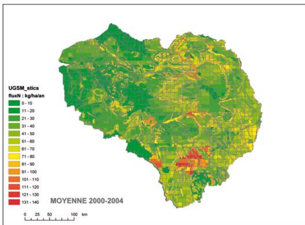
Figure 16 : Flux moyens d'azote sous racinaire (N) calculés par unité de simulation sur le bassin et sur la période 2000/2004 (en kg/ha de SAU/an).
